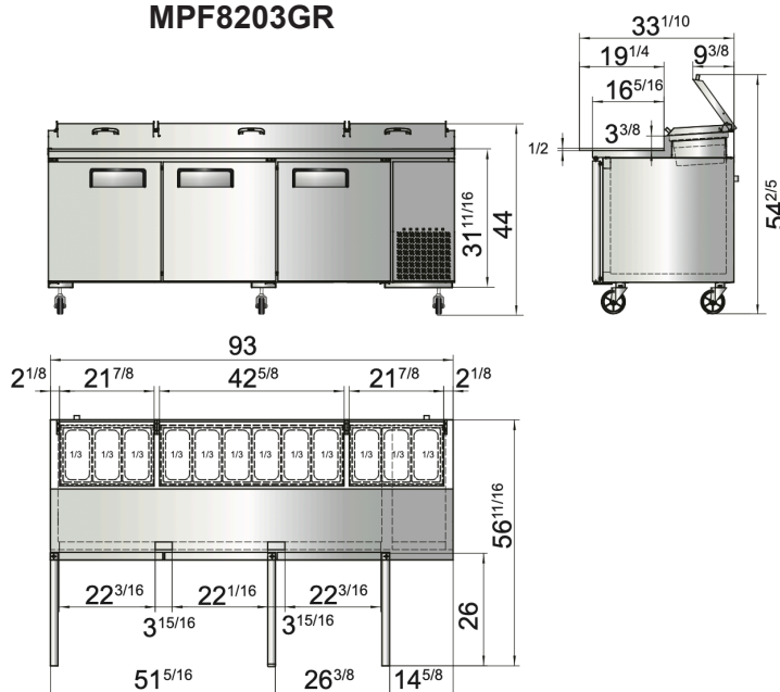
MPF8203GR
