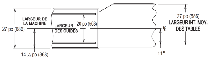
AGENCEMENT PROPOSÉ POUR LES GUIDES ET LES TABLES
