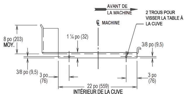
ILLUSTRATION DE LA POSITION DES TROUS DANS LA BORDURE RECOURBÉE DE LA TABLE
