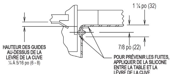
COUPE ILLUSTRANT L'ASSEMBLAGE DES TABLES
